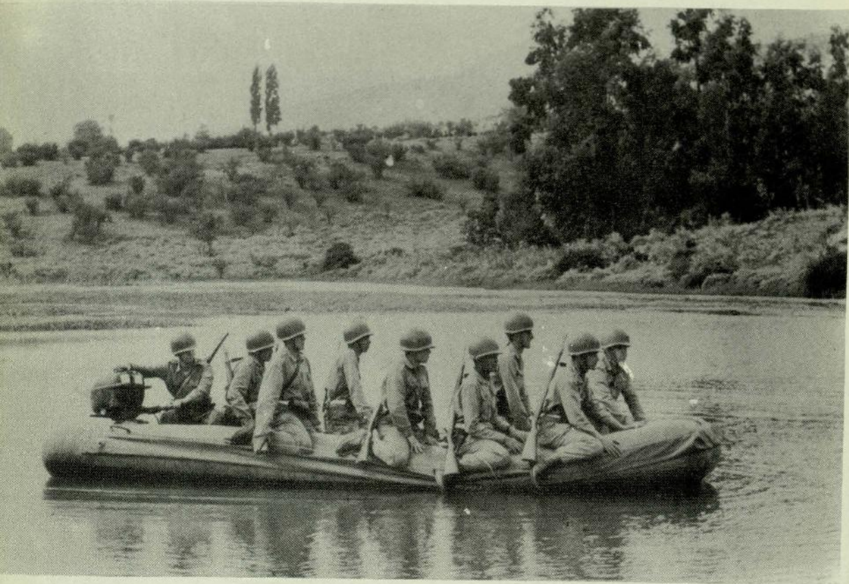
PONTON NEUMÁTICO. — Patrulla de Ingenieros en instrucción de navegación y reconocimiento de cursos de agua, para una posterior construcción de puentes.
