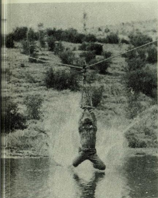
Construcción de pasarelas suspendidas en el área de instrucción de la Escuela, empleando material circunstancial
