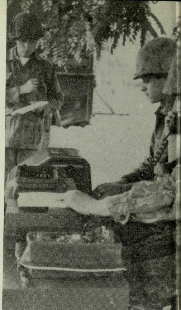
Puesto de Teleimpresores AN-PGC-1 integrando una Central de Telecomunicaciones Adelantada, es operado por alumnos del último curso.
