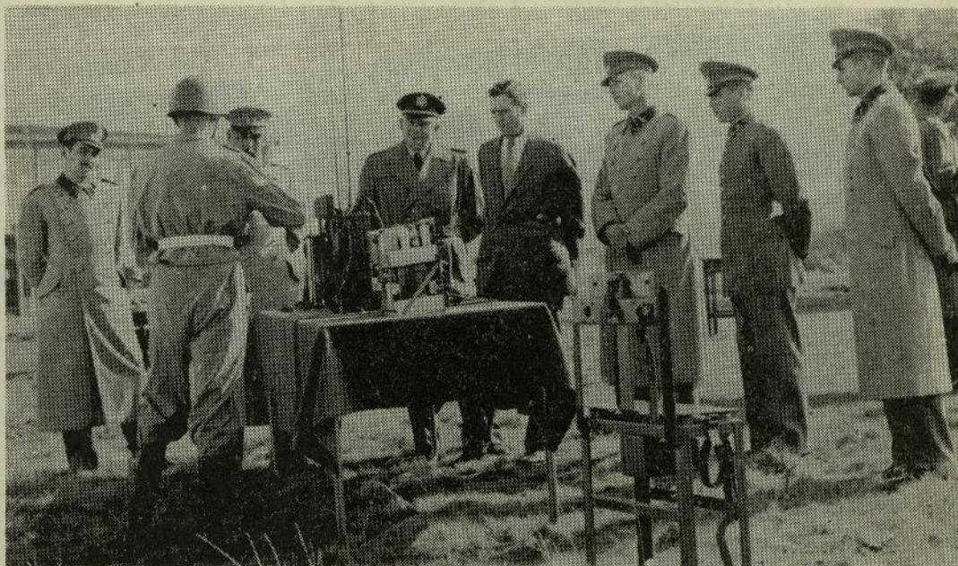
Un Alférez del Arma explica las diferentes etapas que componen el transmisor de un equipo de radio de campaña al señor Coronel Agregado Militar de EE. UU., durante su visita a una instrucción de Telecomunicaciones.
