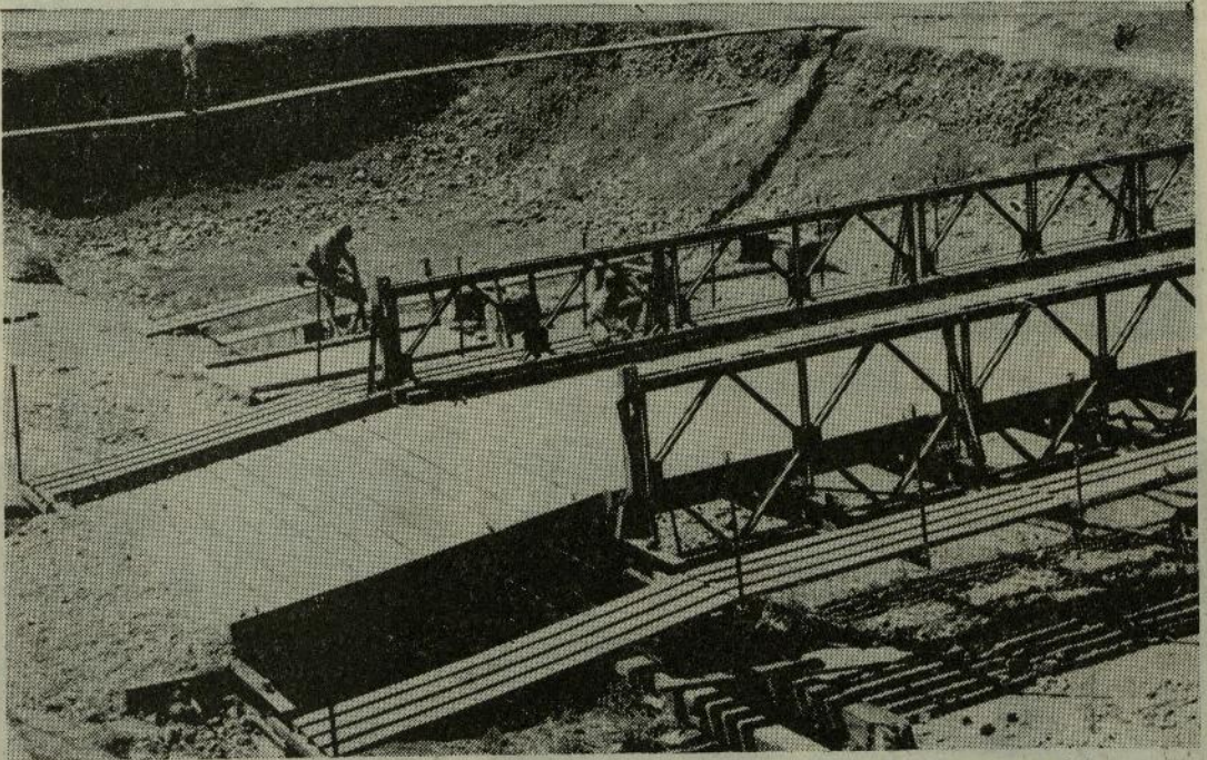
Diferentes medios de pasos construidos durante la Instrucción de Ingenieros del Curso Militar.
