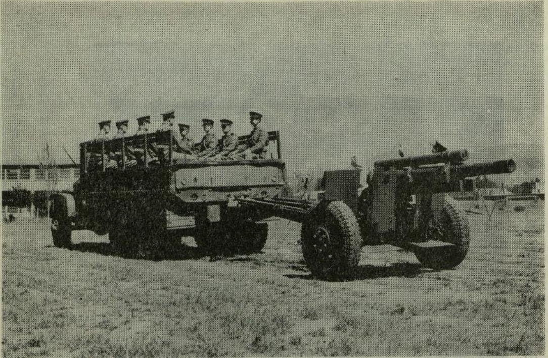
PIEZA PARA EL FUEGO ..... ALTO!! Los Sirvientes y Municioneros de una Pieza 105 mm. N. A. se aprestan a desenganchar la Pieza en la Zona de Posiciones.
