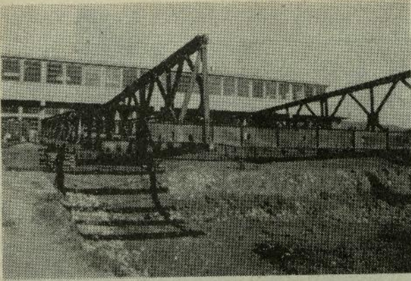
Lanzamiento de un moderno Puente Bailey, sobre la Piscina descubierta de la Escuela.
